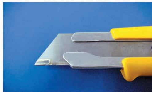
※ 刃先部に超硬チップを接合して成形研削した超硬製替刃です。 (上の写真は市販の大型カッターナイフに超硬製替刃CK-01を装着した状態です。)
